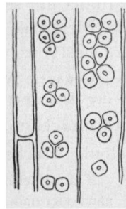
Abb. 2. Protocedroxylon transiens Eckh. Nach Gothan aus Eckhold (7). Radialschnitt. Sterngruppen von Tracheidenhoftüpfeln im Frühholz.
