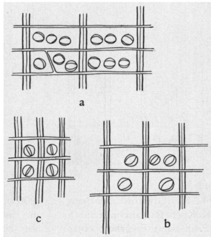
Abb. 12. Sequoia sempervirens Endl. Radialschnitte: a. durch das äusserste Frühholz, b. durch das Folgeholz, c. durch das Spätholz. Taxodioide Tüpfelung.
