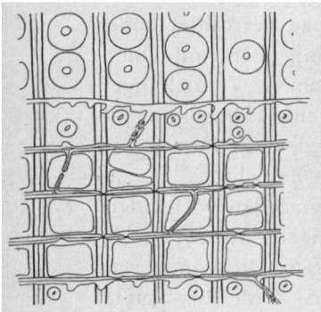
Abb. 7. Pinus laricio . Radialschnitt durch das Frühholz. Quertracheiden mit Zacken. Grosse Eiporen auf den Kreuzungsfeldern; abietoide Tüpfelung der Tracheidenwände, schwach ausgebildete abietineentüpfelung der Markstrahlzellwände.
