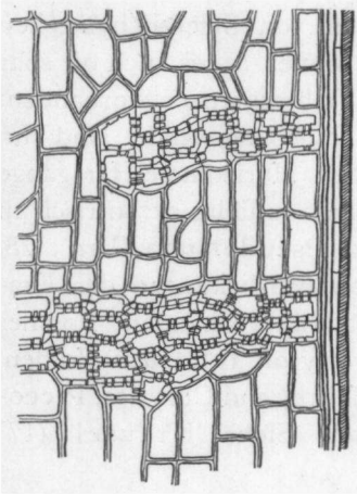
Abb. 9. Picea polita . Radialschnitt durch dem Markkörper eines vierjährigen Astes. Platten von Sklerenchymzellen.
