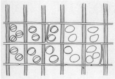
Abb. 13. Glyptostrobus pensilis K. Koch. Radialschnitt durch das Früh- und Folgeholz eines jungen Astes. Glyptostroboide Kreuzungsfeldtüpfelung.
