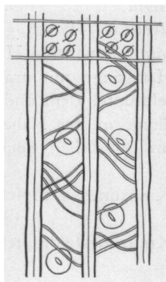
Abb. 4. Torreyia spec. Radialschnitt durch das Frühholz. Spiralige Verdickungen der Tracheidenwände gruppenweise angeordnet. Kreuzungsfeldtüpfel mit lang ausgezogenen Poren.
