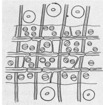
Abb. 18. Thuja occidentalis L. Radialschnitt durch das Frühholz. Typisch cupressoider Tüpfelung. Verdickte Markstrahlquerwände und sehr dünne tangential Markstrahlzellwände.
