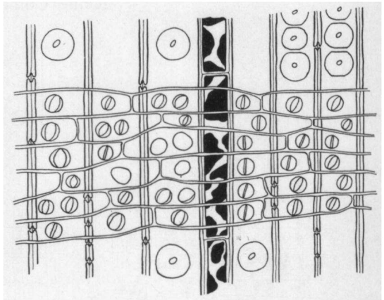
Abb. 14. Podocarpus Beccari . Radialschnitt im Bereich einer Jahresgrenze, die von der mit Harz gefüllten Holzparenchymzellenreihe gebildet wird. Einige Hoftüpfel ein wenig abgeplattet. Podocarpoide Kreuzungsfeldtüpfelung.
