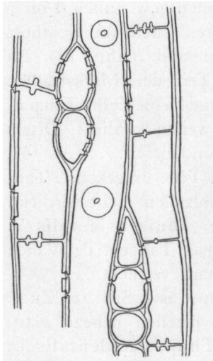
Abb. 19. Taxodium distichum Rich. Tangentialschnitt durch das Frühholz. Verdickungsknoten auf den Querwänden der Holzparenchymzellen.
