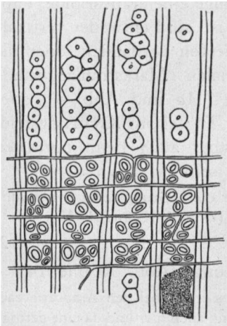
Abb. 1. Araucaria imbricata . Radialschnitt durch das Frühholz. Araucarioide Tüpfelung, Tracheide mit Harzfällung.
