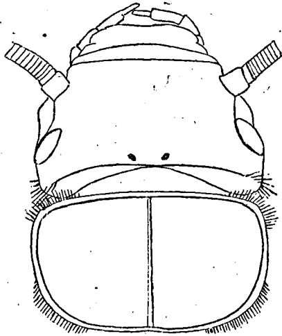
Fig. 1. Neoperla spec. A.—Nymphe.
