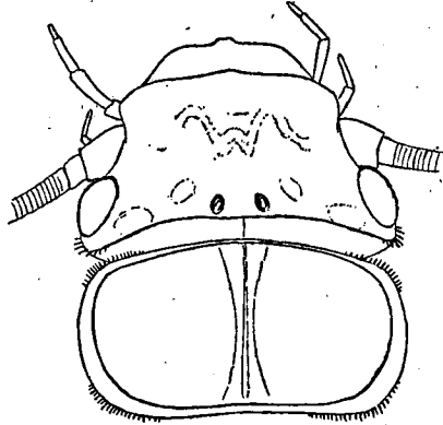
Fig. 2. Neoperla spec. B.—Nympha.
